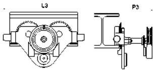
Modelo HTP 500 - 5,000 kg con guía de cadena de mando giratoria y topes de goma
