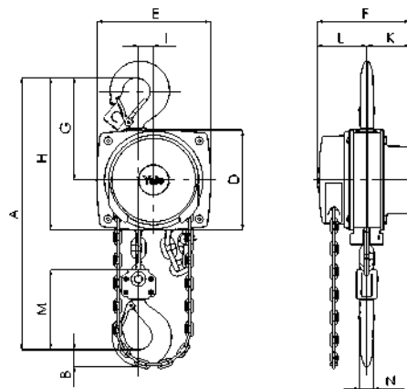
Modelo Yalelift 360/500 - 3,000 kg, un ramal
